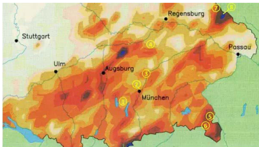
Bodenkontamination im Jahr 1986 in Teilen Bayerns und Baden-Württembergs. Je dunkler markiert ein Gebiet, desto höher mit Cs-137 belastet. Die Ziffern geben Probeentnahmeorte an. (Bild: BFS)
